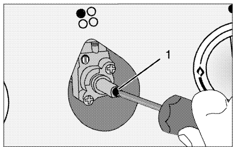
1 Gasdurchfluss-Einstellschraube
